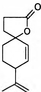
2a 5R, 8S b 5S, 8S
